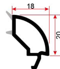
7027 ÇİFT CAM ÇİTASI DOUBLE GLAZING BEAD
