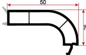
2807 ÇİFT CAM ÇITASI (24 mm) DOUBLE GLAZING BEAD (24 mm)
