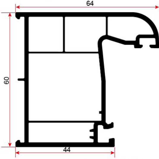
6023 PENCERE KANAT PROFİLİ SASH PROFILE
