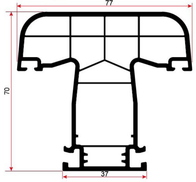
6004 KAPI KANAT PROFİLİ DOOR SASH PROFILE
