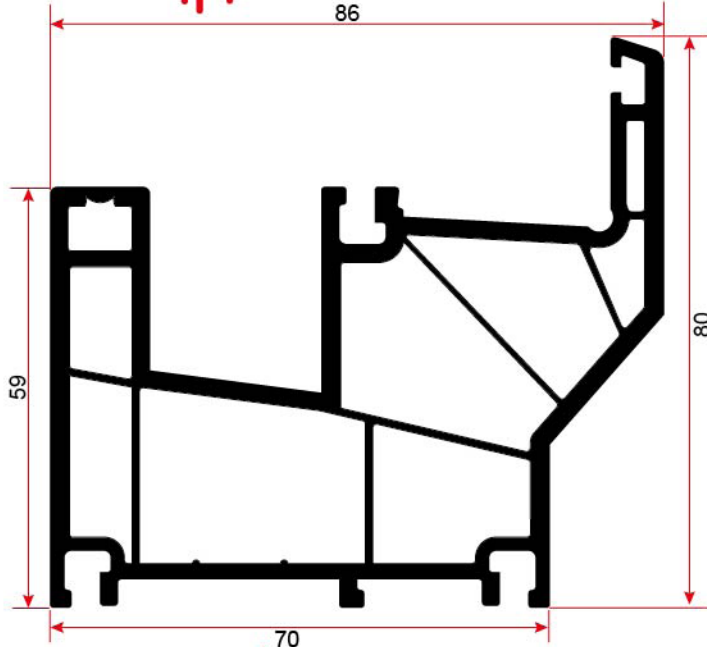
8002 SÜRME PERVAZLI KASA SILL DOUBLE FRAME PROFILE
