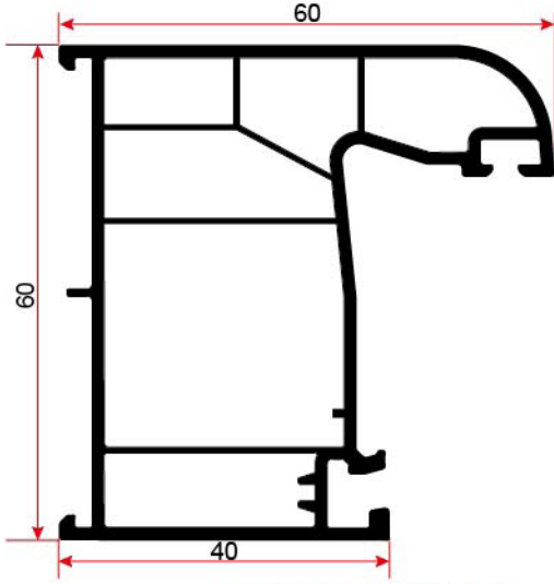
6003 PENCERE KANAT PROFİLİ SASH PROFILE
