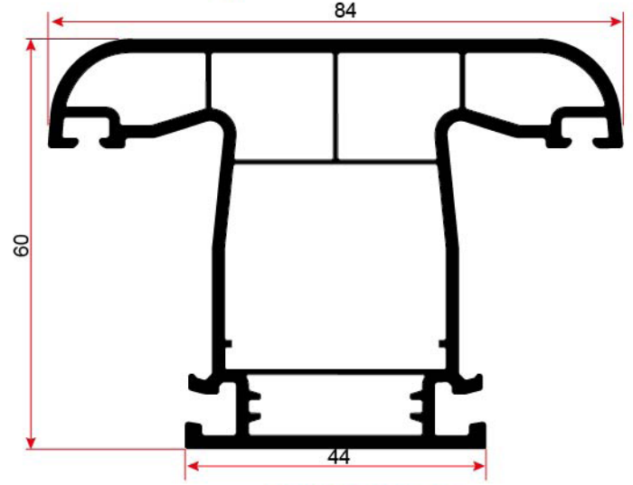
6024 KAPI KANAT PROFİLİ DOOR SASH PROFILE
