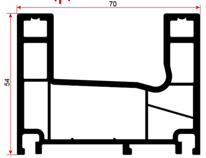
8001 SÜRME ÇİFTLİ KASA PROFİLİ DOUBLE FRAME PROFILE
