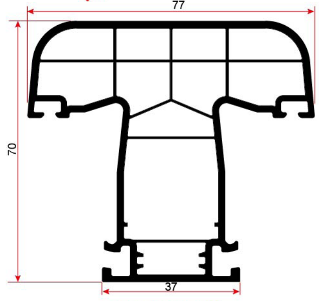
6024 KAPI KANAT PROFİLİ DOOR SASH PROFILE
