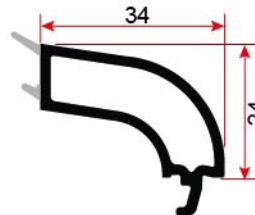
2807 ÇİFT CAM ÇITASI (24 mm) DOUBLE GLAZING BEAD (24 mm)
