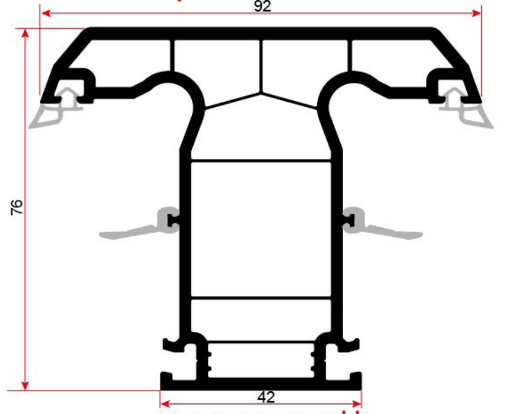
2204 KAPI KANAT PROFİLİ DOOR SASH PROFILE
