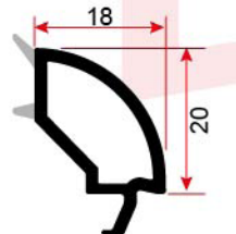
7027 ÇİFT CAM ÇITASI (34 mm) TRIPLE GLAZING BEAD (34 mm)
