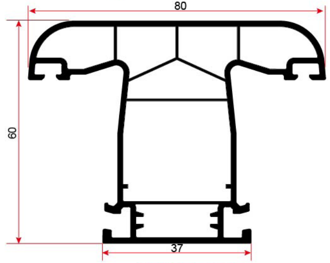
6004 KAPI KANAT PROFİLİ DOOR SASH PROFILE
