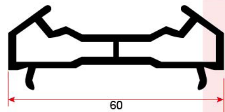
9002 KÖŞE DÖNÜŞ ADAPTÖRÜ CORNER TURNING ADAPTER
